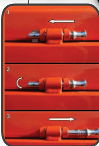
Nowy układ łączników pomiędzy pierwszą a drugą burtą
